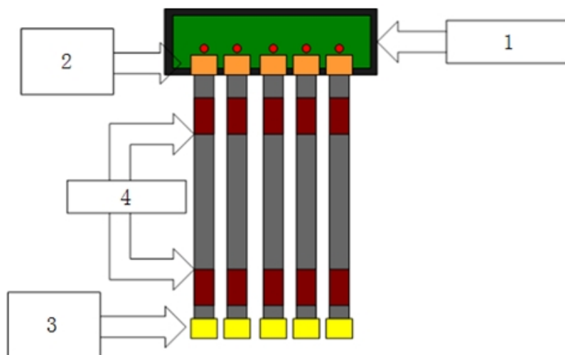
钢带监测装置结构简图
